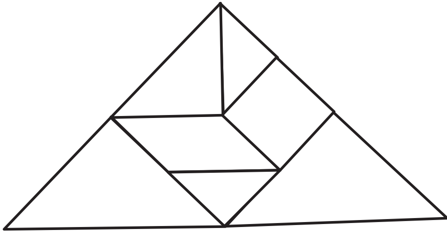
직각이등변삼각형
